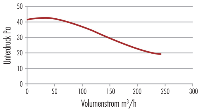
Leistungsdiagramm AirSpeedy®
